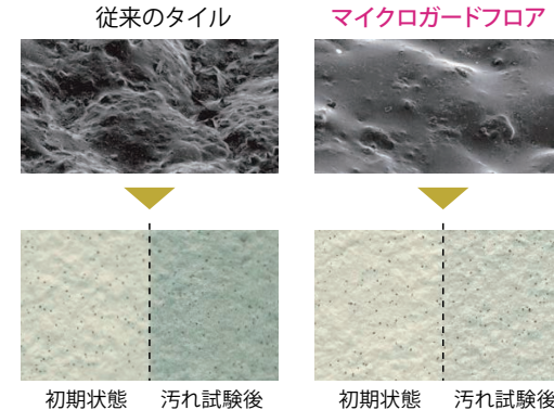
LIXIL 独自の厳しい汚れ試験(強制汚れ試験)を実施しました。マイクロガードフロアは汚れのつき方が少なく明確な差が出ました。
